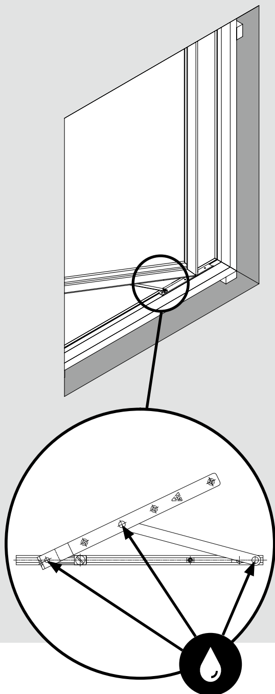
Schwingfenster Sidestyrt vindu Sidestyret vindue Okno uchylne boczne Side Slide window Sidohängt fönster med glidbeslag Taatsraam
