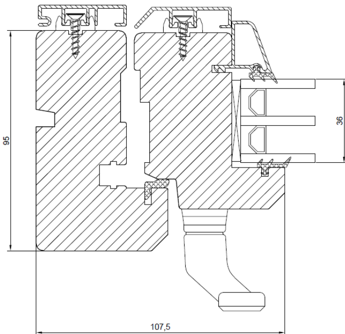
Sidestycke med handtag Sidestykke med håndtak Side with handle
